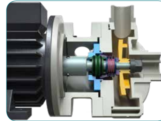
TS = Gleitringdichtung
